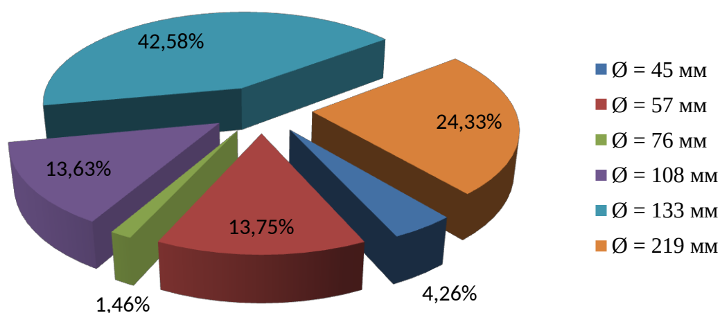
Рисунок 2.3.2.2 – Доли протяжённости участков трубопроводов тепловых сетей котельных ООО «Компания теплоснабжения» различных диаметров
