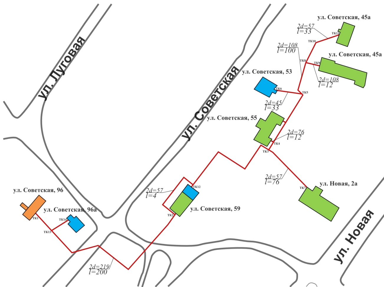
Рисунок Б – Карта-схема тепловых сетей ООО «Компания теплоснабжения» в зоне действия котельной, с. Большая Шелковка
