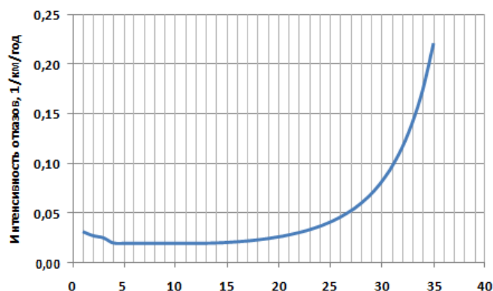
Рисунок 8.1 – Интенсивность отказов в зависимости от срока эксплуатации участка тепловой сети
