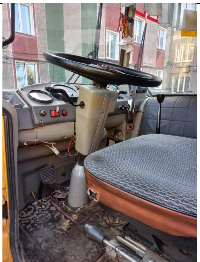
ПАЗ-32053, Место водителя
